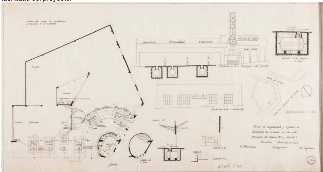
(Fig. 7) Planta, sección y alzados. E.1/100. Archivo Subirana.
